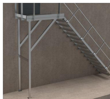
FIXATION AU SOL PAR PIÈTEMENTS
